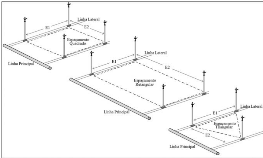
Figura 10. Espaçamento quadrado, retangular e triangular dos aspersores.
