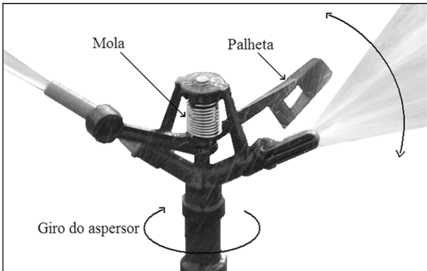
Figura 8. Detalhe da “palheta” que é acionado pelo impacto do jato d’água.
