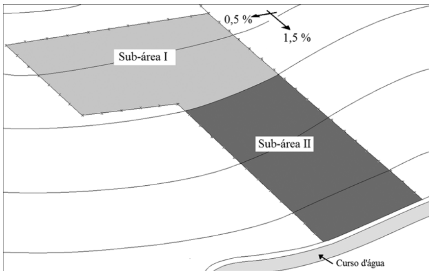
Figura 74. Subdivisões da área.
