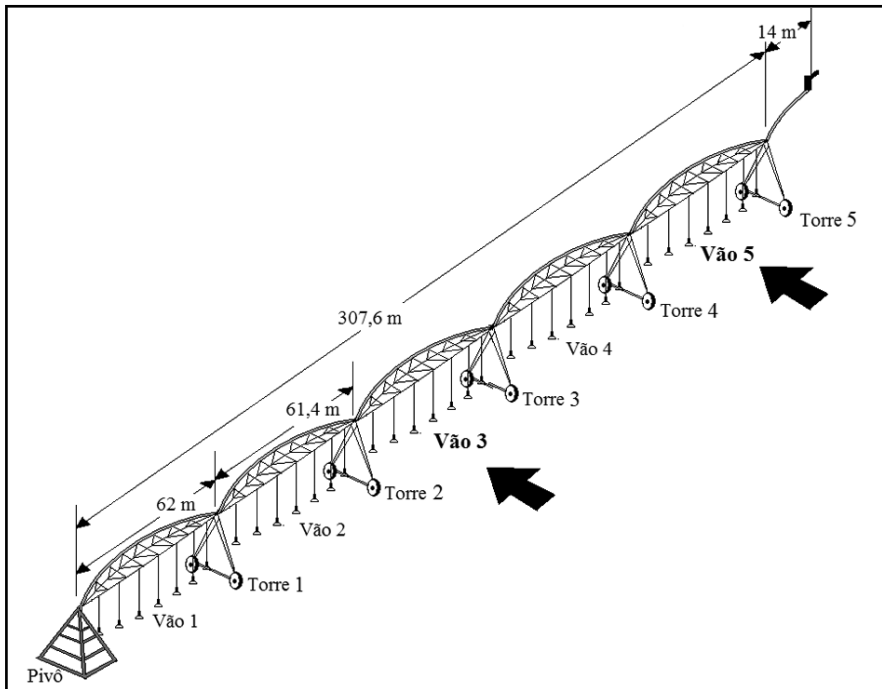
Figura 32. Aplicação prática: dimensões do pivô central.
