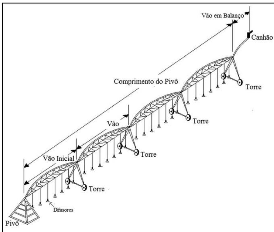
Figura 31. Esquema de um pivô central.
