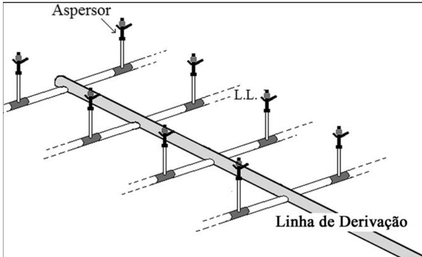
Figura 18. Linha de derivação.
