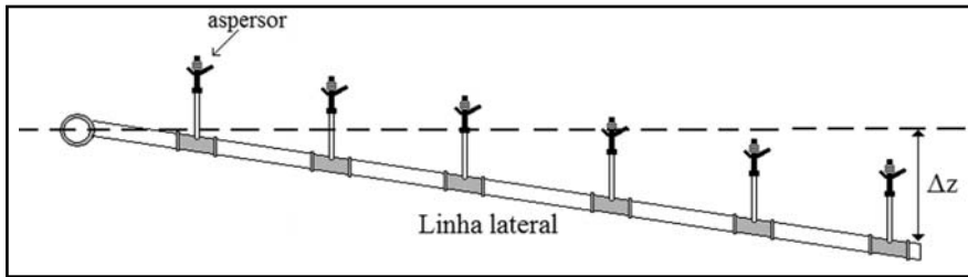
Figura 17. Linha lateral em declive.
