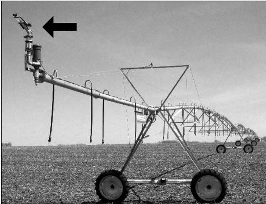
Figura 30. Canhão. (Fonte: http://www.generalirrigation.com/ )
