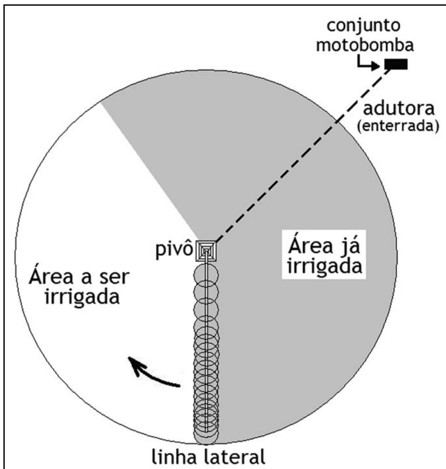
Figura 27. Área irrigada pelo pivô.
