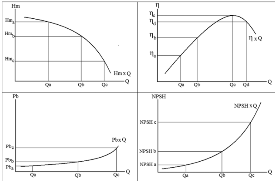
Figura 71. Curvas características.
