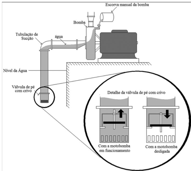
Figura 70. Escorva manual da bomba.
