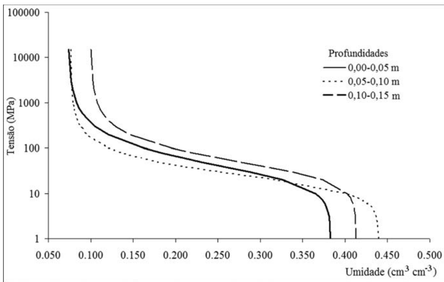
Figura 44. Curvas de retenção para cada faixa de profundidade do solo.
