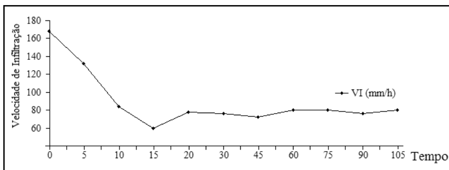
Figura 55. Velocidade de infiltração.
