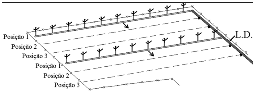
Figura 78. Linhas laterais operando simultaneamente.
