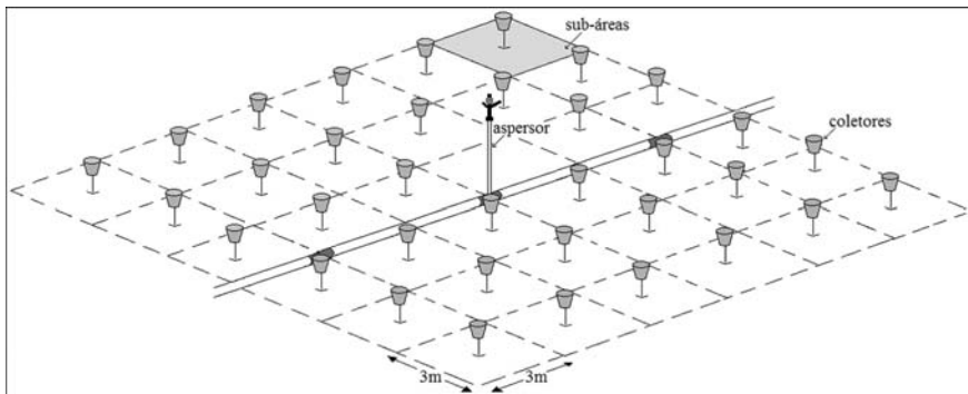
Figura 60. Coletores colocados no centro de cada subárea.
