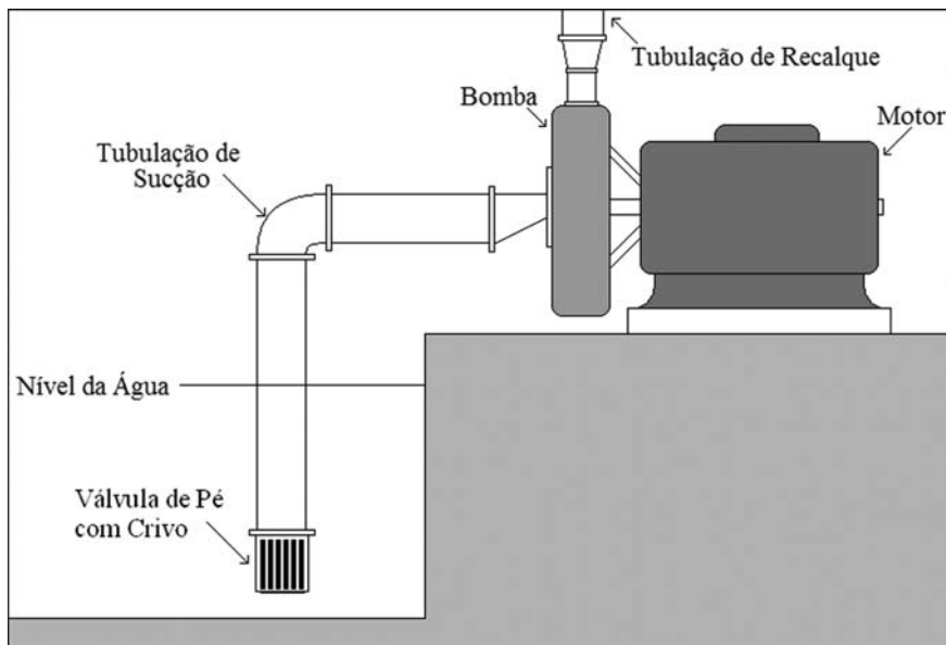
Figura 13. Conjunto motobomba.
