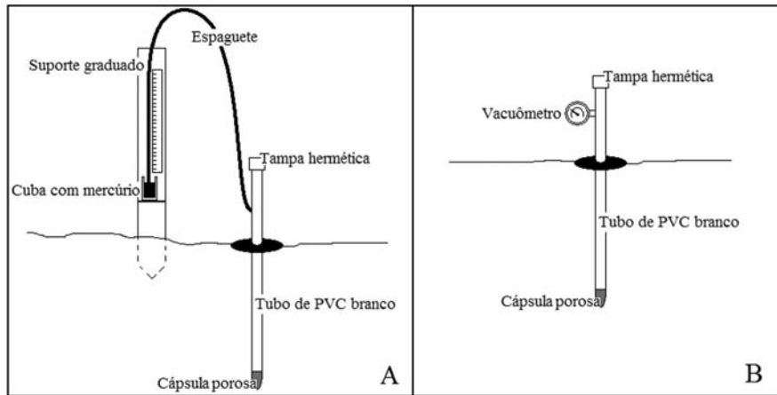
Figura 43. Tensiômetro de mercúrio e de vacuômetro.
