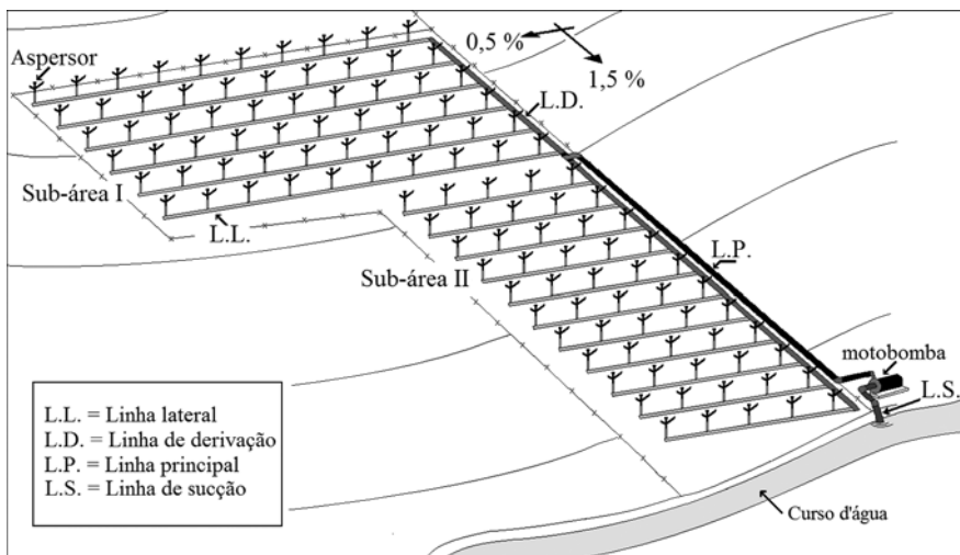
Figura 75. Distribuição do equipamento no campo.
