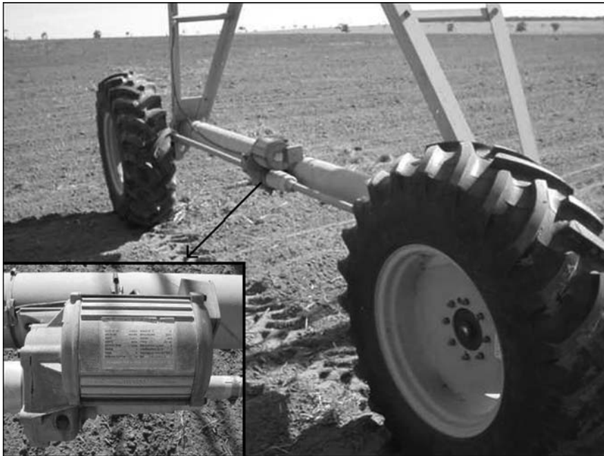
Figura 24. Rodas e motor de uma torre.
