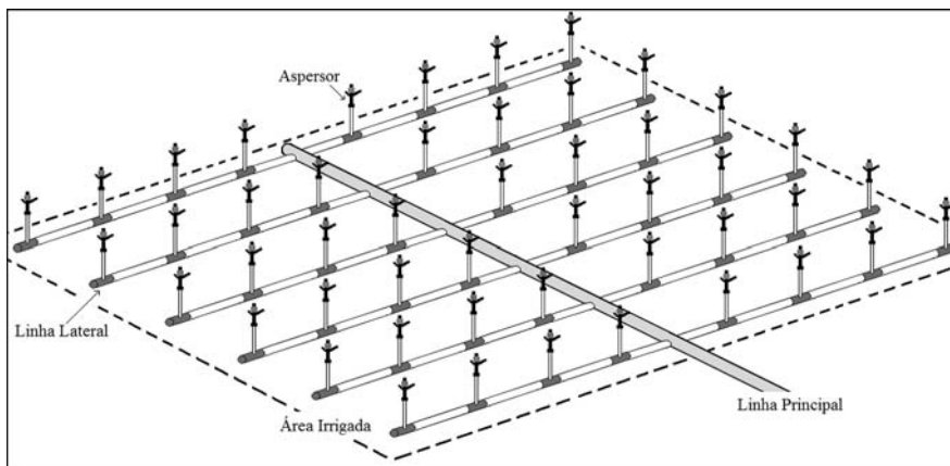
Figura 3. Sistema convencional permanente.
