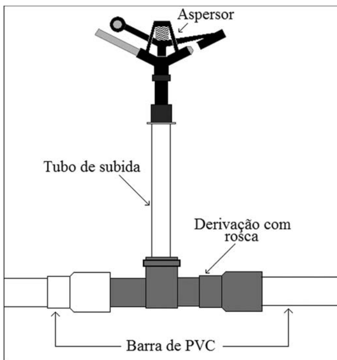
Figura 76. Aspersor, derivação com rosca e tubo de subida.
