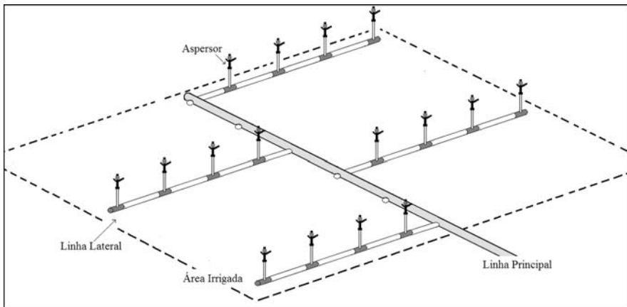
Figura 2. Sistema convencional portátil de irrigação.
