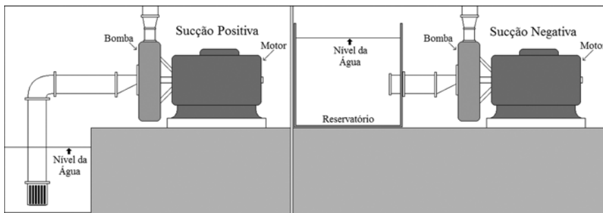
Figura 69. Sucção positiva e negativa.
