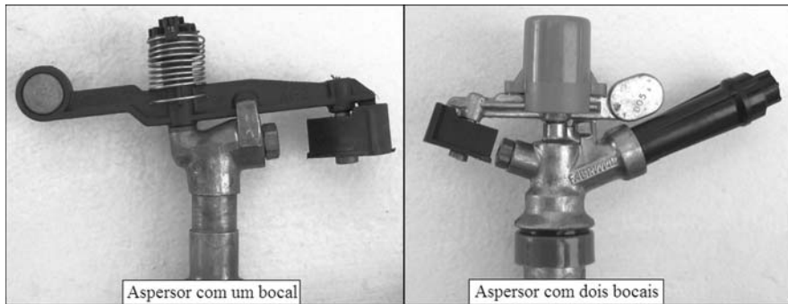
Figura 7. Aspersores com um e dois bocais.
