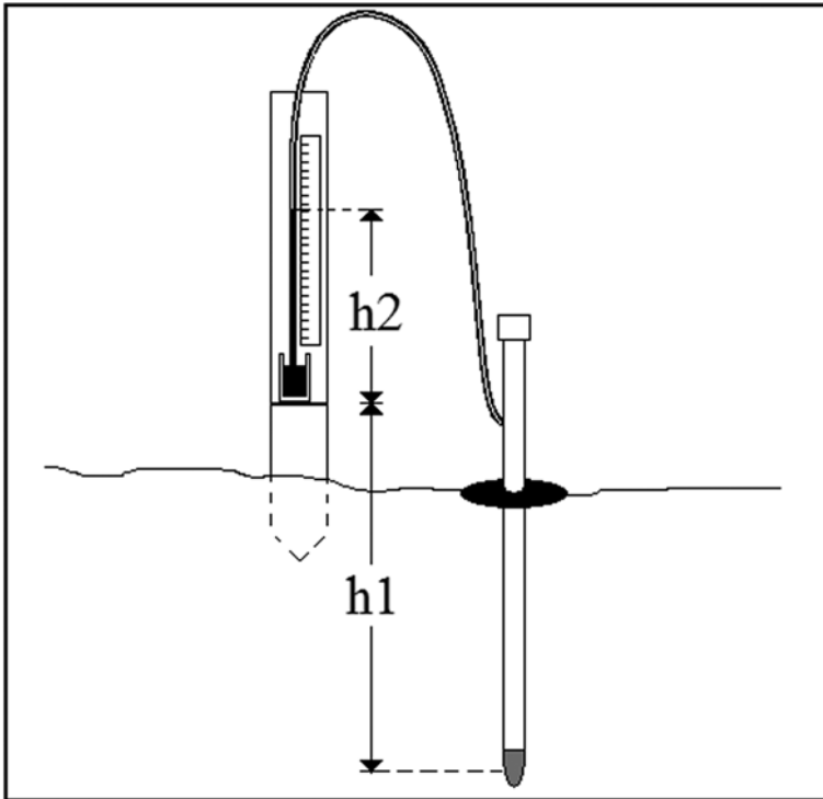
Figura 43. Tensiômetro de mercúrio.
