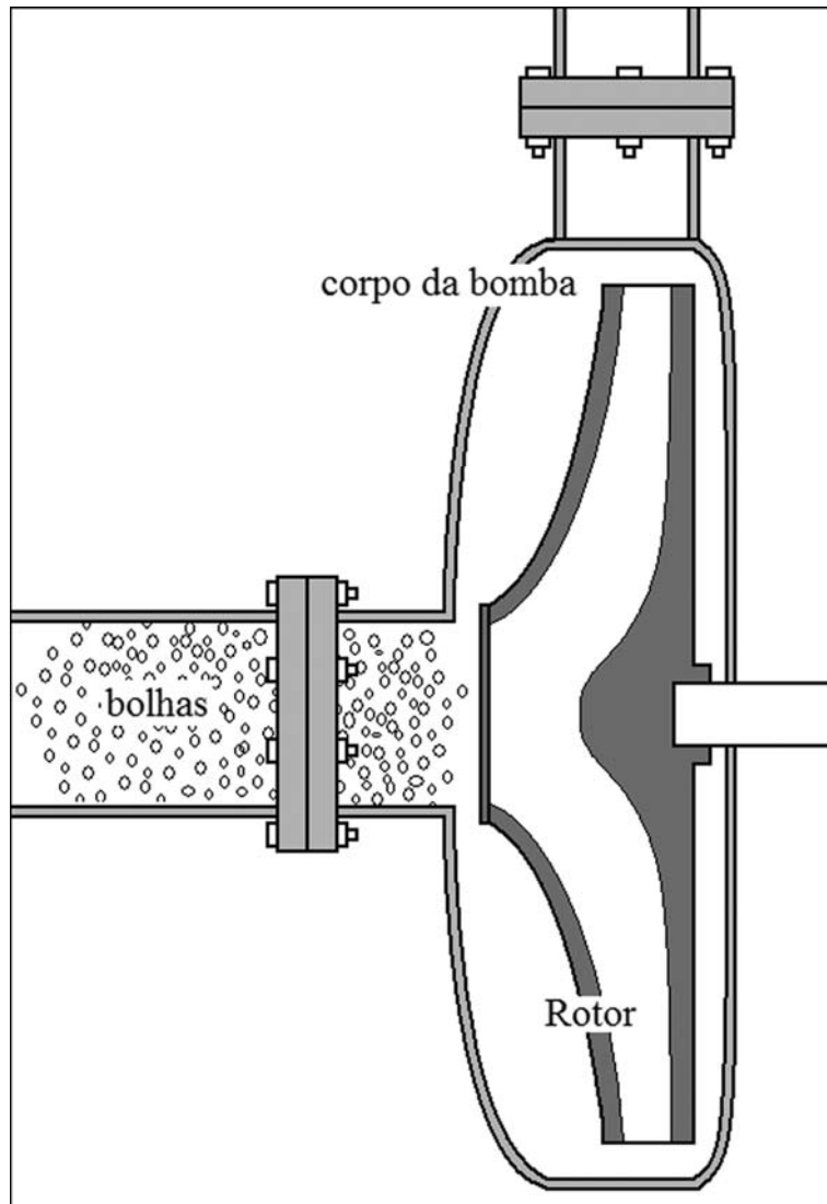
Figura 72. Cavitação.
