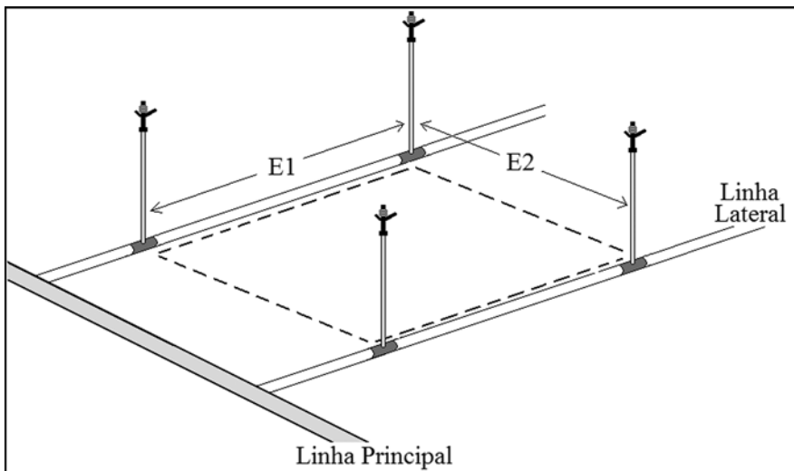
Figura 9. Espaçamento entre aspersores.
