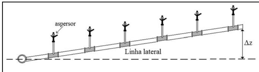
Figura 16. Linha lateral em active.
