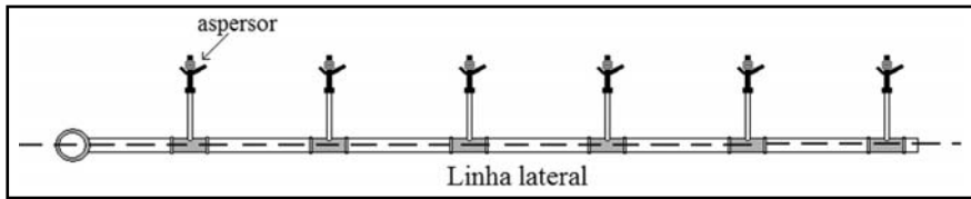
Figura 15. Linha lateral em nível.
