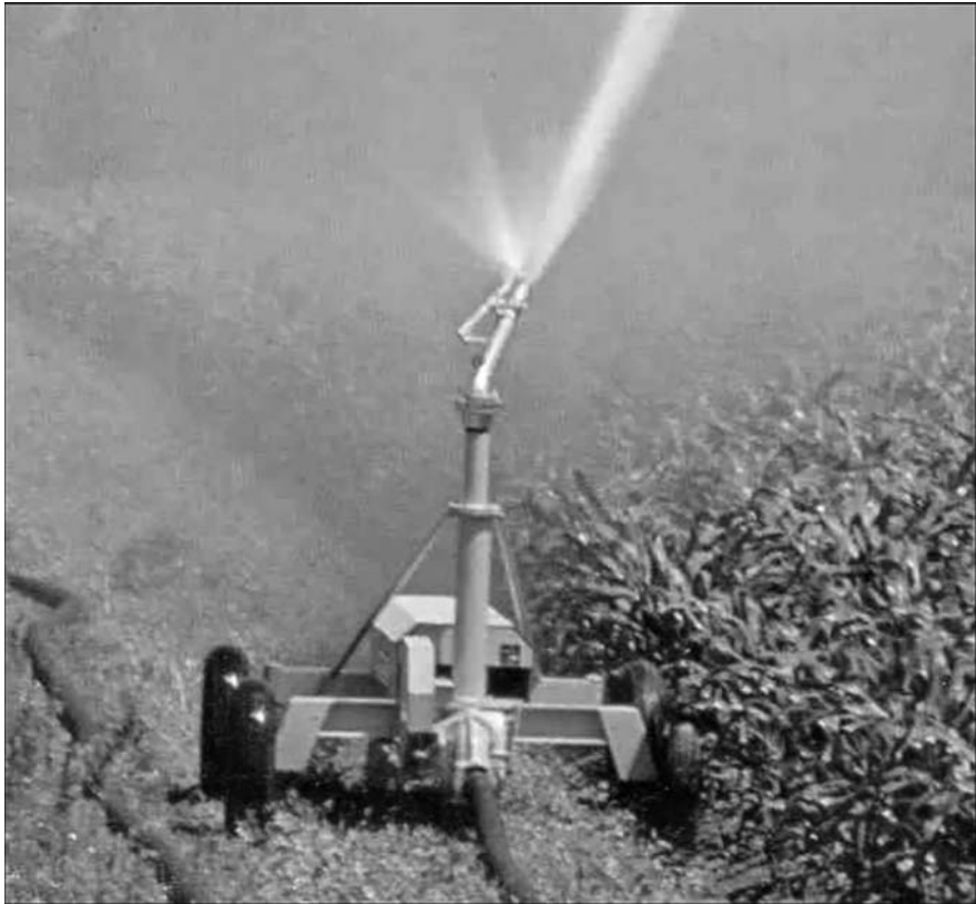
Figura 36. Autopropelido. (Fonte: www.clemson.edu/irrig/Equip/Trav.htm )
